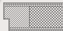
Einbruchhemmende Türen, stumpf 70-RC2-SK3 mit Zusatzfalz
