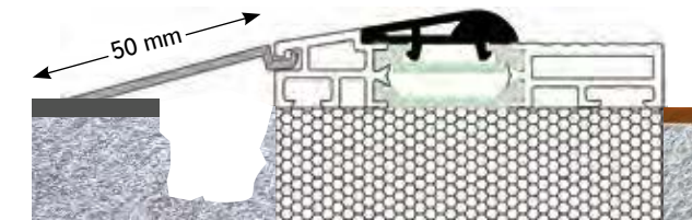
Flachbodenschwelle Spezial mit zusätzlicher Anschlussblende
