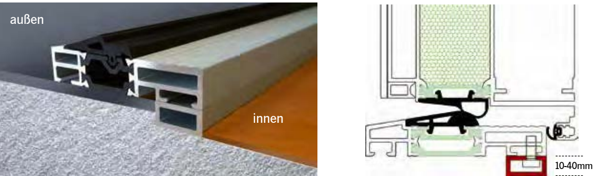
Aluminium-Rechteckrohr auf der Innen- und/oder Außenseite an Tür und Seitenteil; wahlweise innen und/oder außen bündig. Lieferbare Höhen 10, 15, 20, 25, 30, 35 oder 40 mm.
