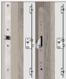
Dreifachverriegelung mit Rundbolzen oder Schwenkhaken
